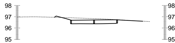
PRZEKRÓJ POPRZECZNY 12+50.84
